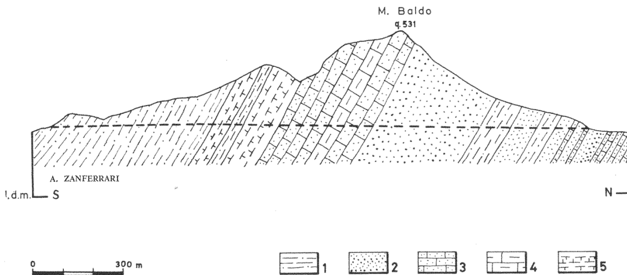
fig. 5 — Sezione geologica semplificata, subparallela all'asse delle gallerie, la cui proiezione sul piano della sezione è indicata dalla linea tratteggiata. 1 - argille e argille siltose; 2 - arenarie generalmente micaceo-glauconitiche, a grana variabile; 3 - calcareniti; 4 - calcari argillosi; 5 - marne.
